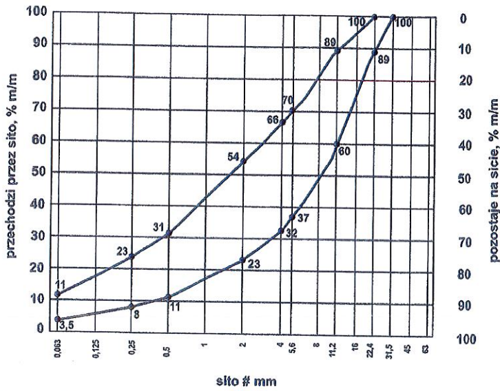
Rys. 2. Krzywe graniczne uziarnienia mieszanki zawiązanej spoiwem drogowym typu 2 o uziarnieniu 0/22,4 mm
